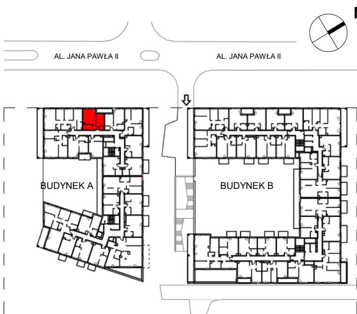
SCHEMAT LOKALU MIESZKALNEGO NA 4 PIĘTRZE
