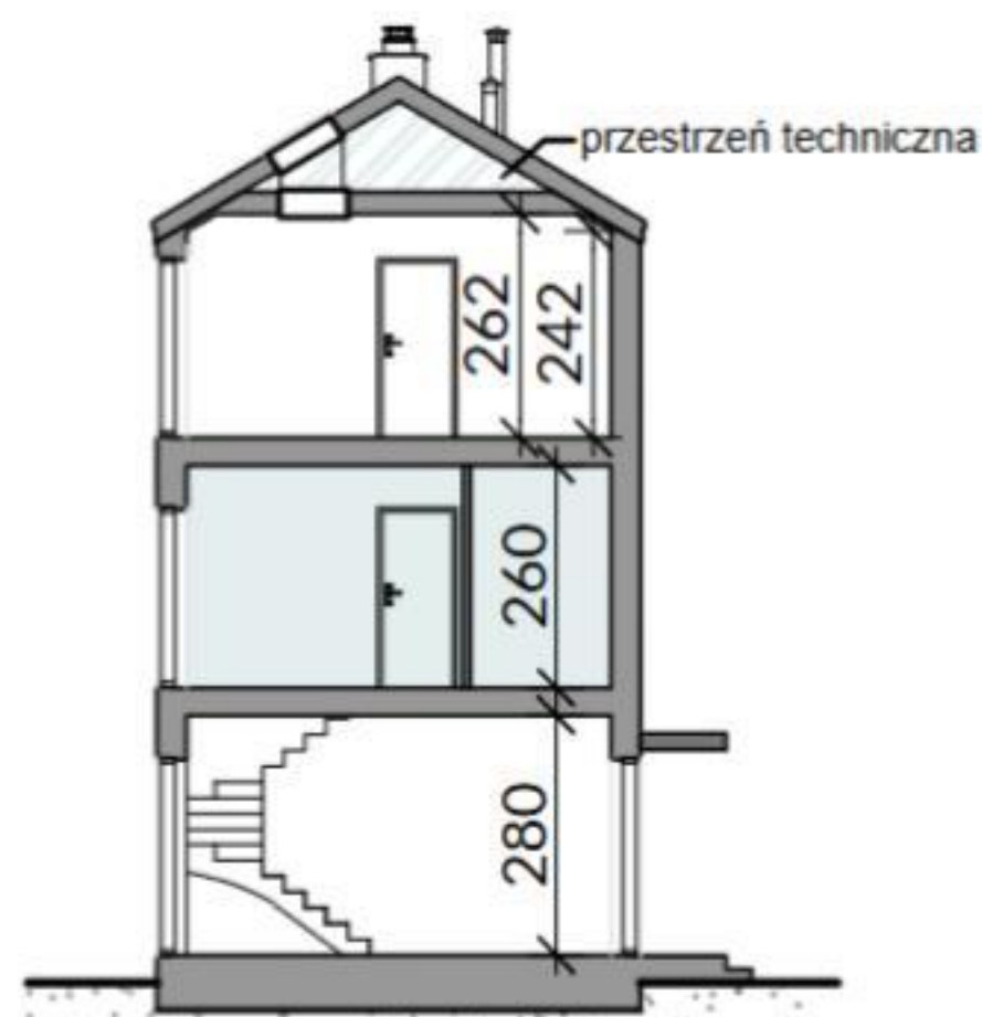
SCHEMATYCZNY PRZEKRÓJ PRZEZ LOKAL
