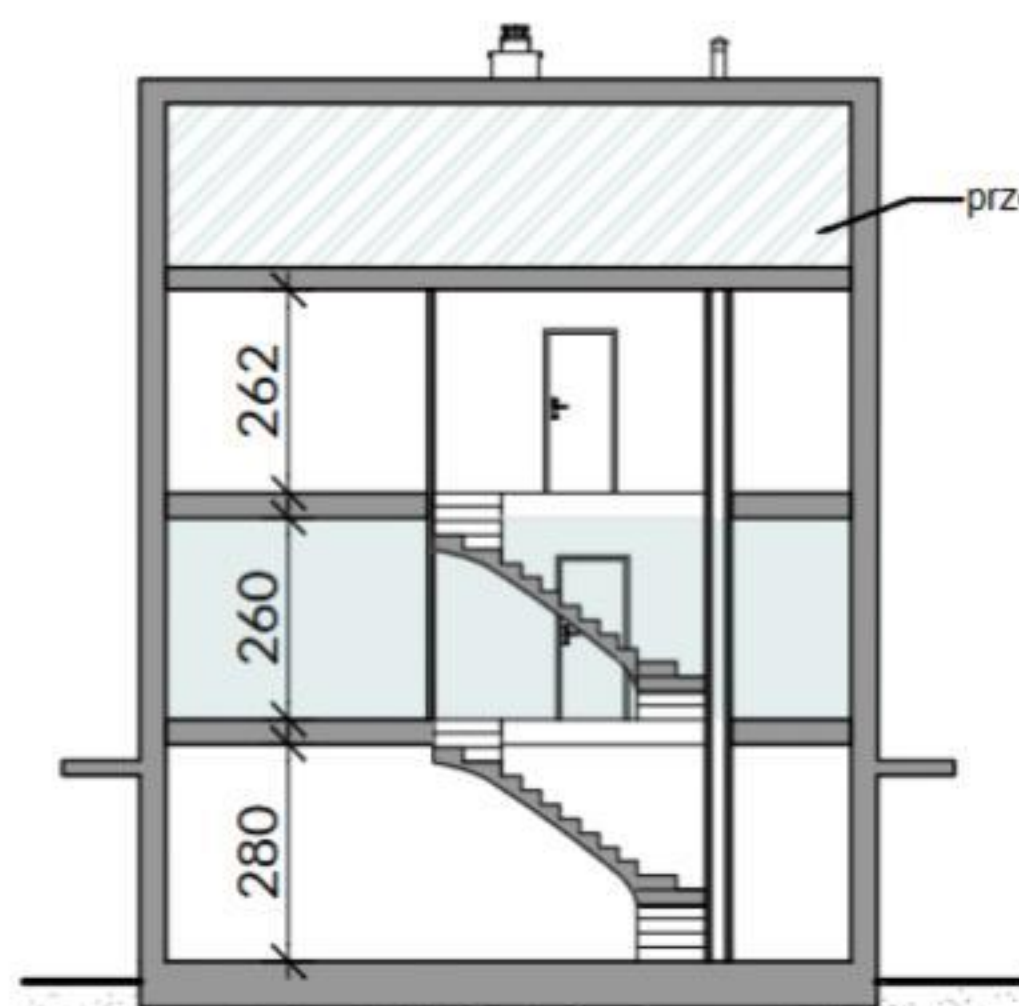
SCHEMATYCZNY PRZEKRÓJ PRZEZ LOKAL
