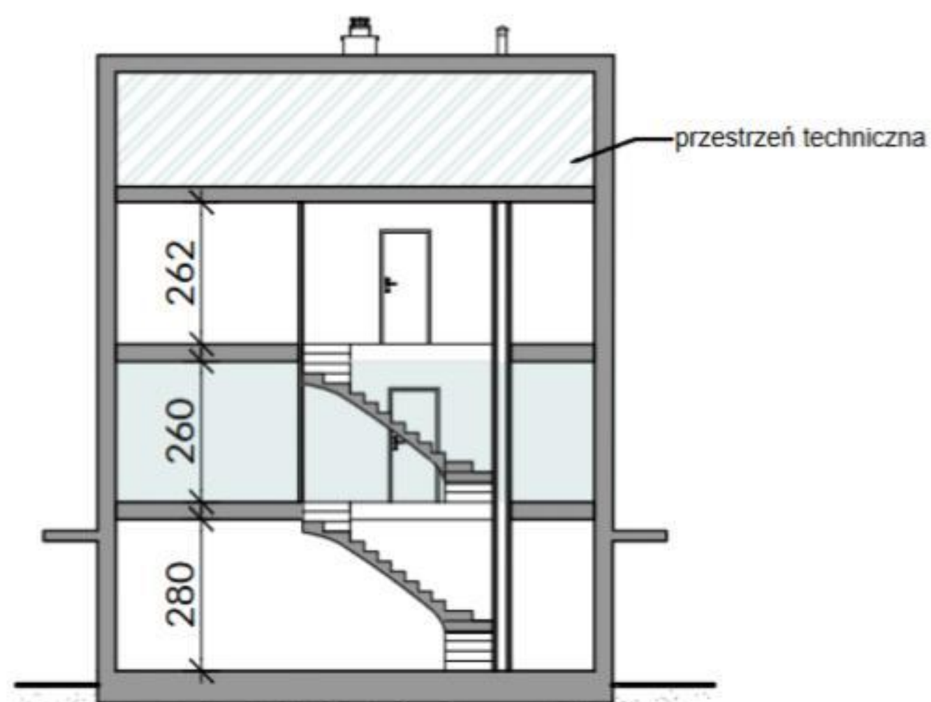
SCHEMATYCZNY PRZEKRÓJ PRZEZ LOKAL
