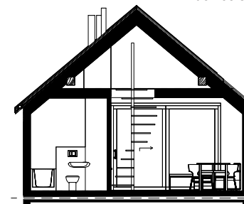
Przekrój poddasza nieużytkowego - 21,25 m 2 podłogi
