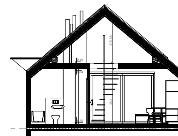
Przekrój poddasza nieużytkowego - 22,33 m 2 podłogi
