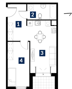
Rzut lokalu
