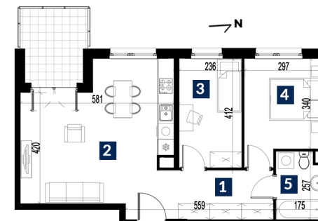
Rzut lokalu
