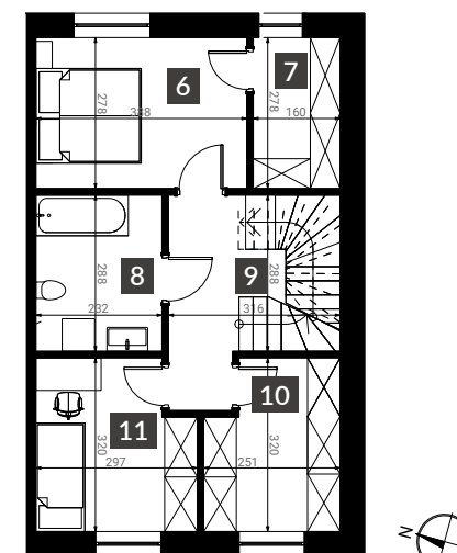
Rzut piętra
