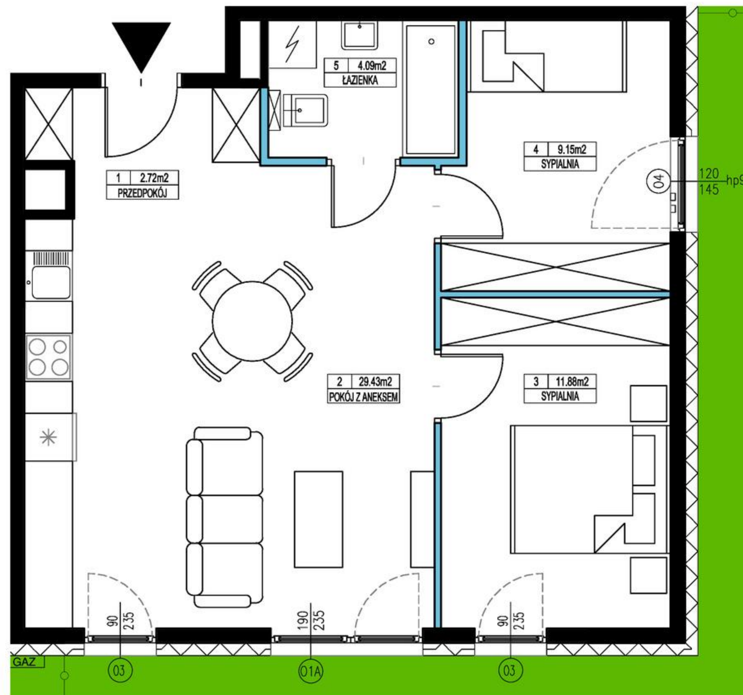
RZUT LOKALU
