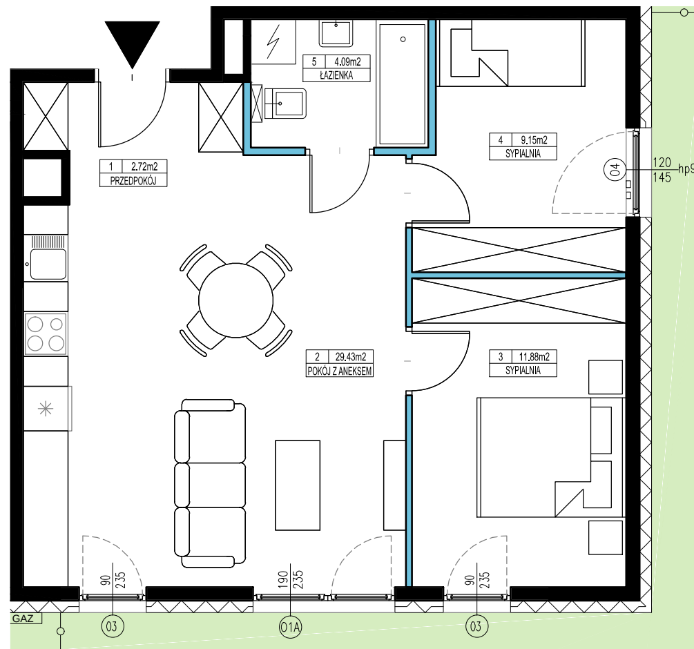
RZUT LOKALU
