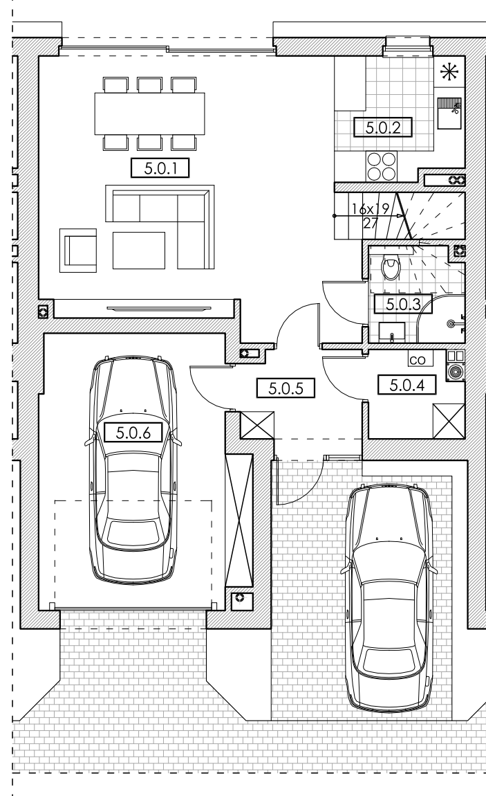
PARTER SKALA 1:100
