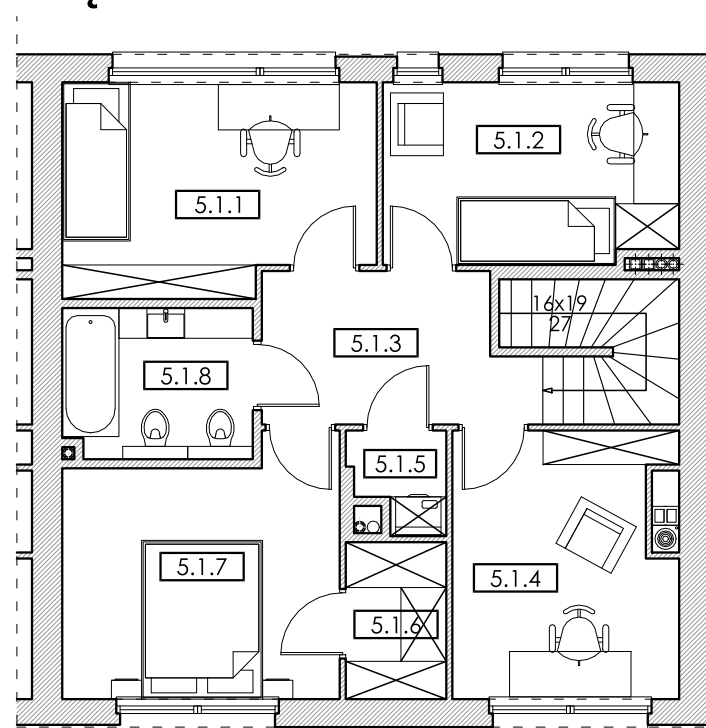
PIĘTRO SKALA 1:100
