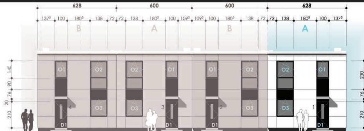
ELEWACJA FRONTOWA
